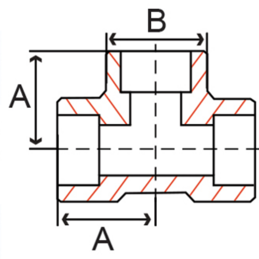
Fig. 52T 3 - Tee
